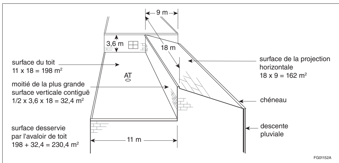
Figure 1-1 Surface de toit à desservir (exemple 1)
