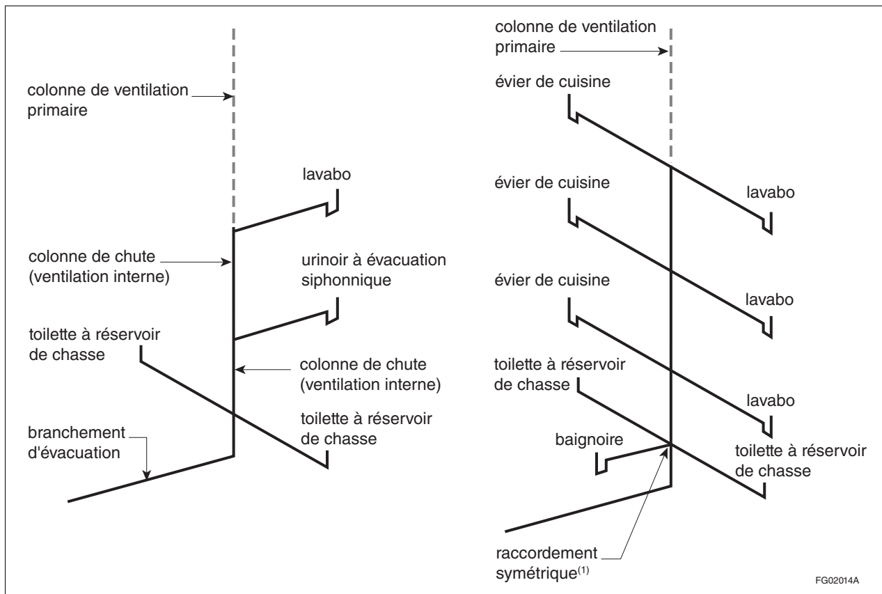
Figure A-2.5.2.1.-B Exemple de ventilation interne décrite à l'alinéa 2.5.2.1. 1)c)
