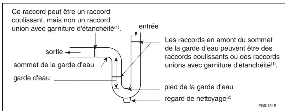
Figure A-2.2.3.1. 1) et 3) Garde d'eau et raccords de siphon
