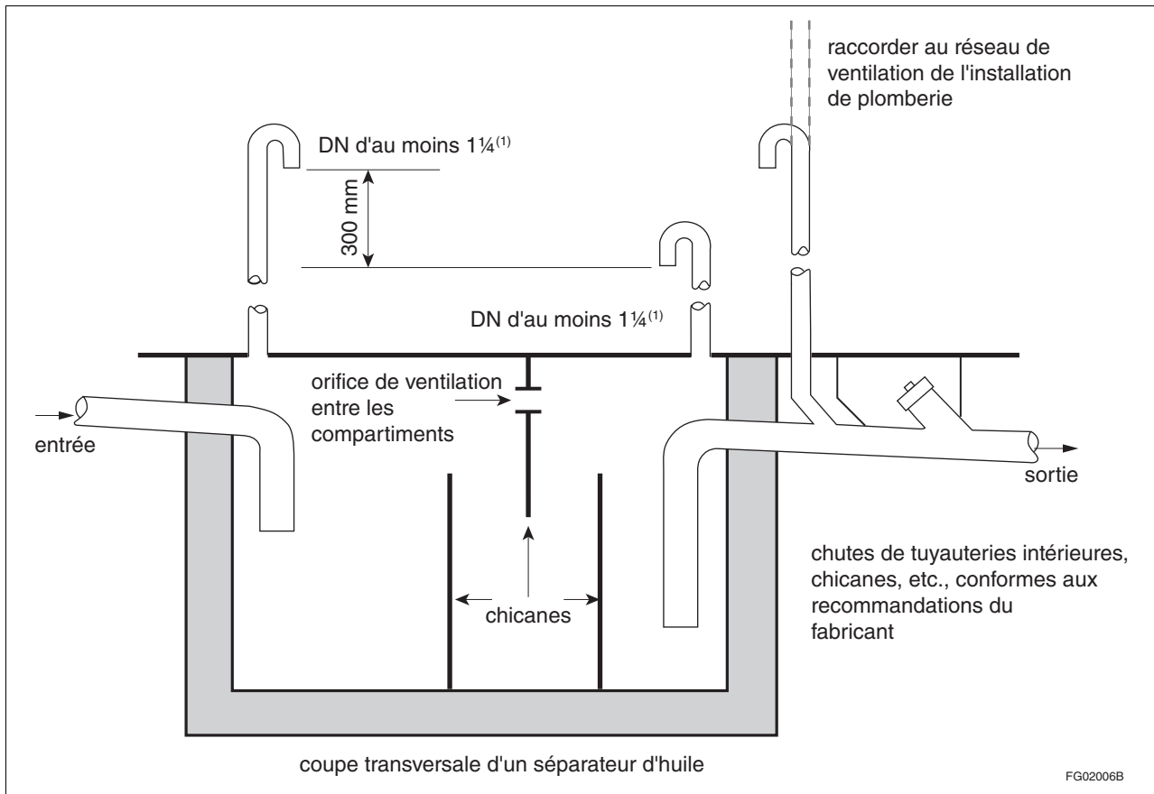
Figure A-2.5.5.2. Séparateurs d'huile
