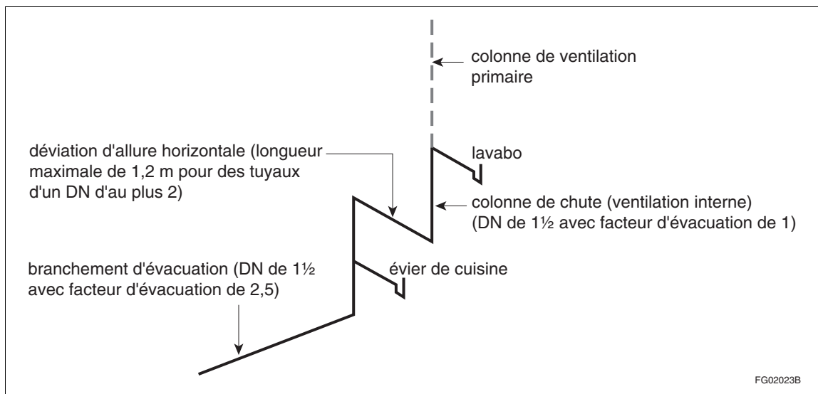
Figure A-2.5.2.1.-J Exemple de ventilation interne décrite au sous-alinéa 2.5.2.1. 1)i)i)
