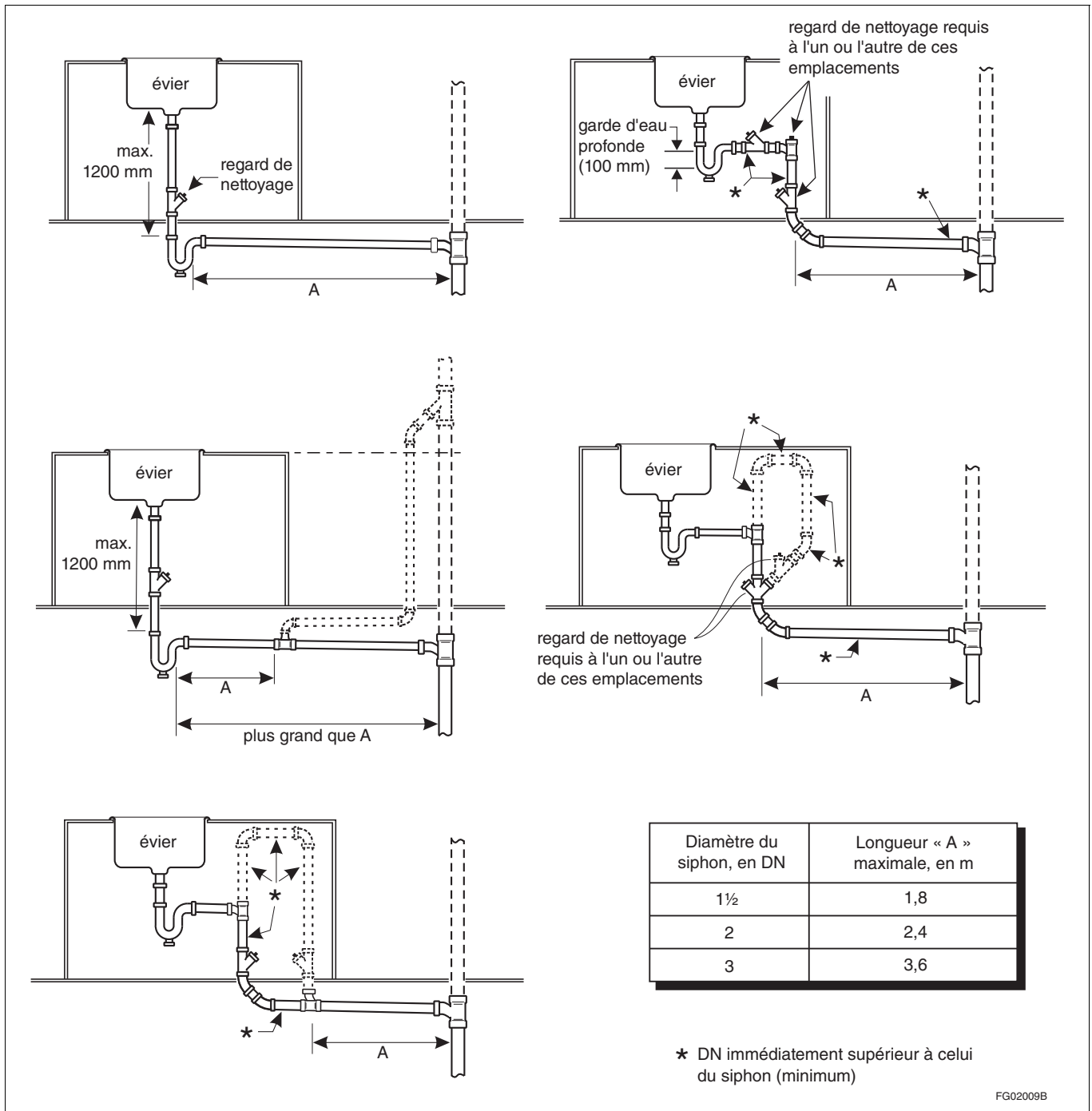
Figure A-2.4.8.2. 1) Installation des appareils sanitaires des meubles îlots
