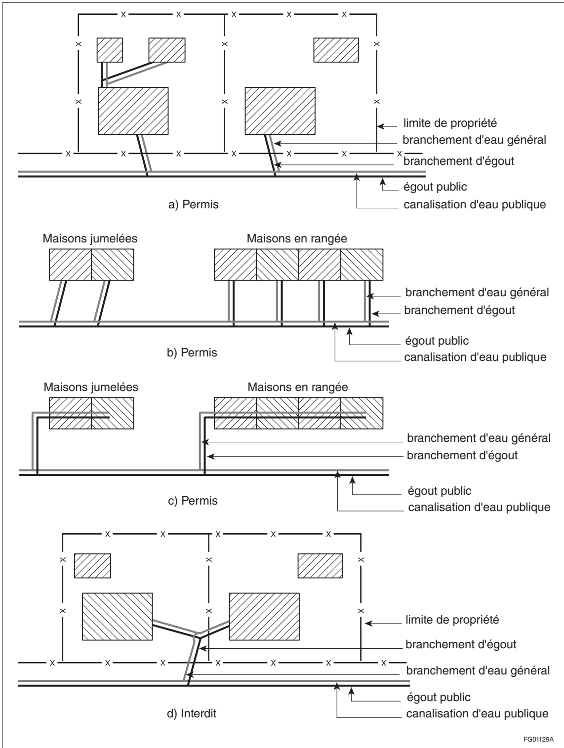
Figure A-2.1.2.4. 1) Raccordement aux réseaux publics
