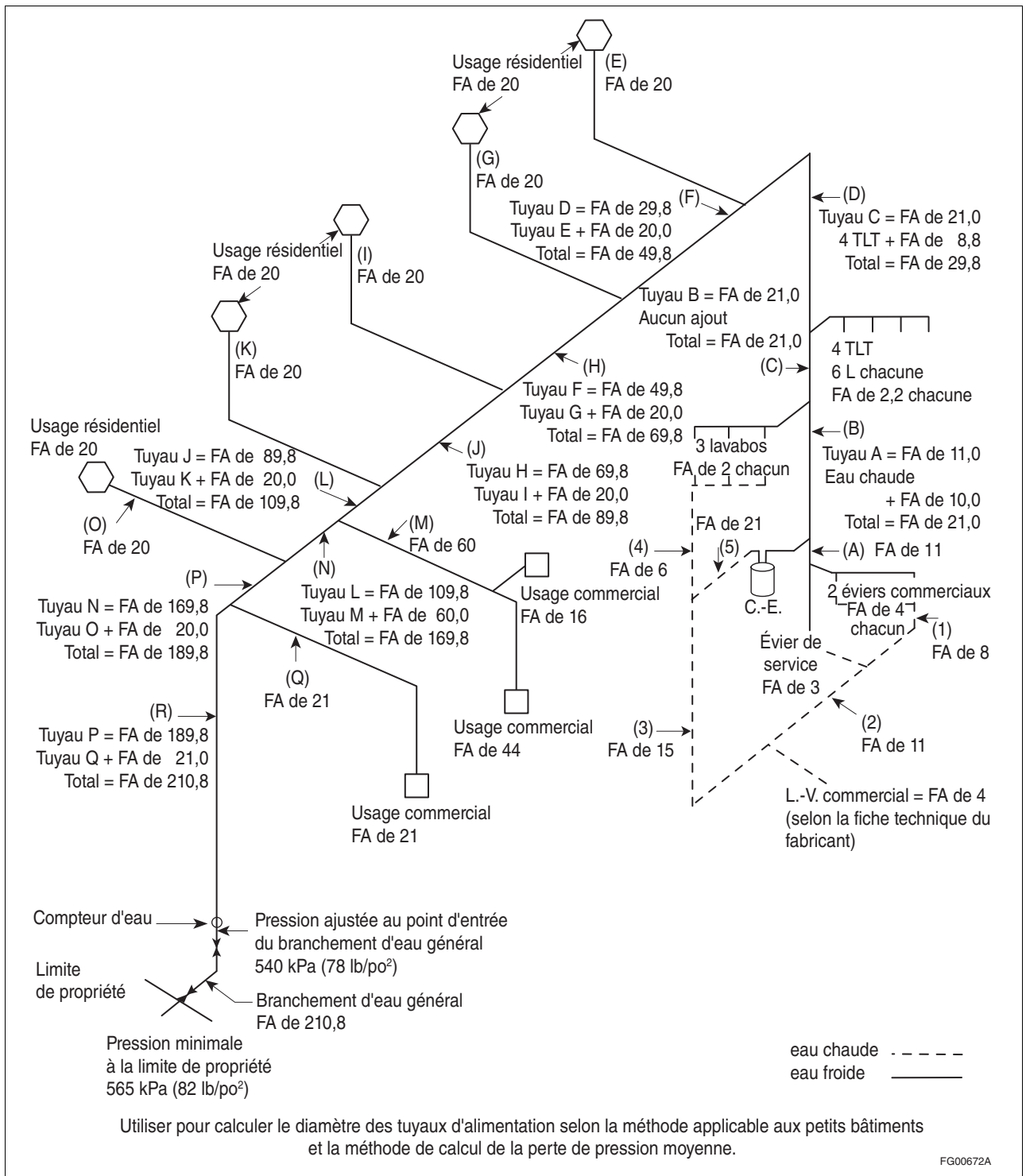
Figure A-2.6.3.1. 2)-A
