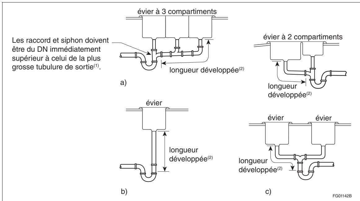
Figure A-2.4.5.1. 2) Siphons d'éviers et de bacs à laver
