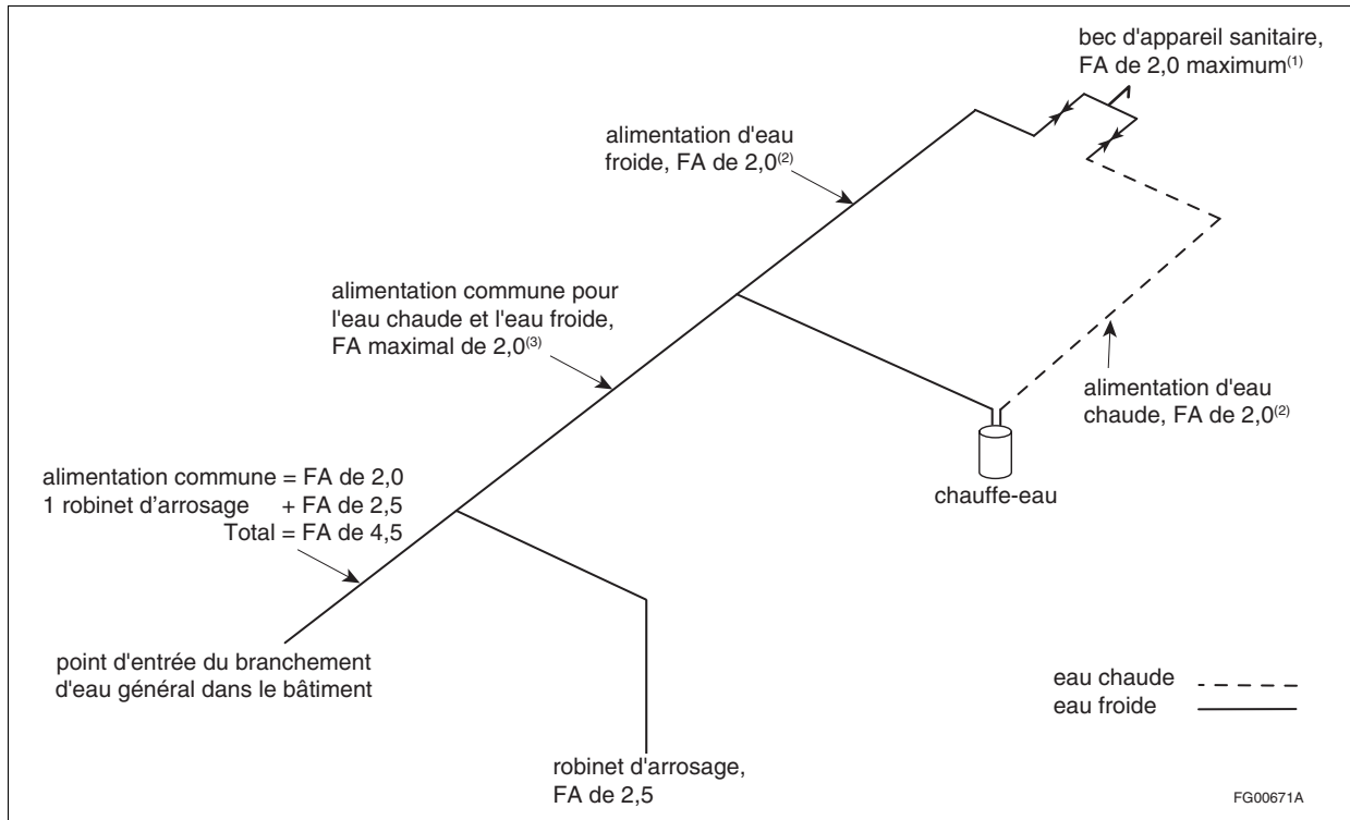
Figure A-2.6.3.4. 5)-A
