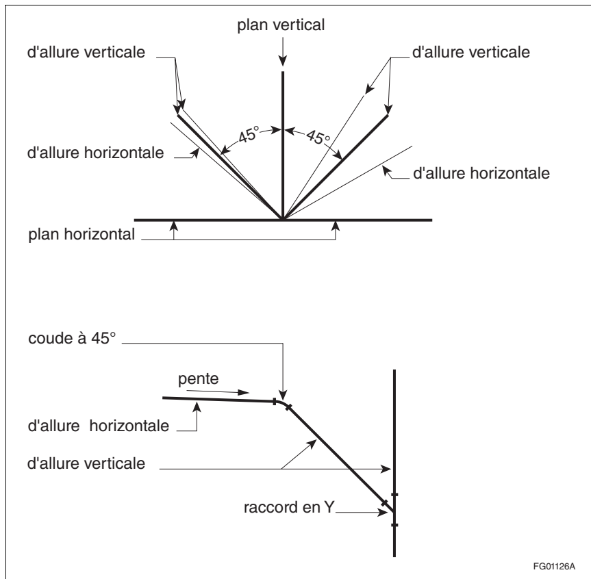
Figure A-1.4.1.2. 1)-D D'allure horizontale et d'allure verticale
