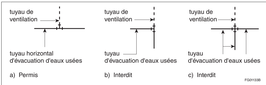
Figure A-2.2.4.1. Utilisation des tés dans les réseaux d'évacuation
