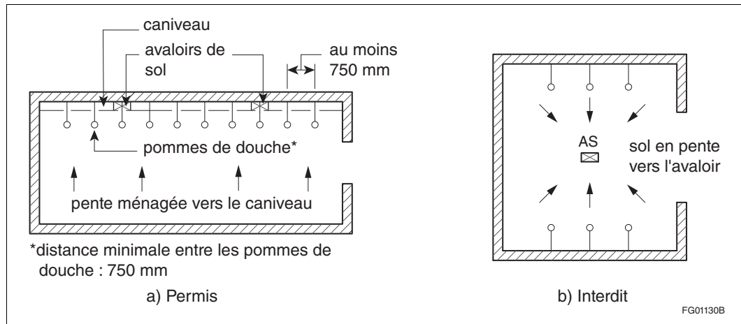
Figure A-2.2.2.3. 3) Évacuation de l'eau des douches (vue en plan)
