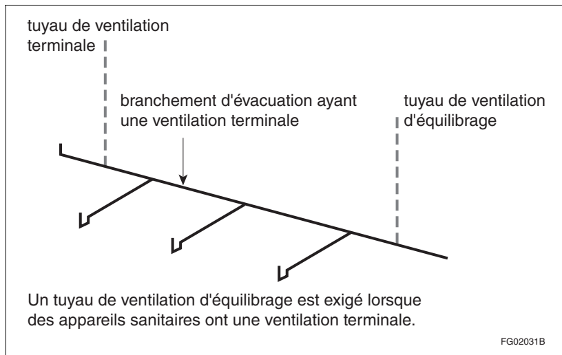
Figure A-2.5.3.1.-D Exemple de ventilation terminale décrite au paragraphe 2.5.3.1. 3)
