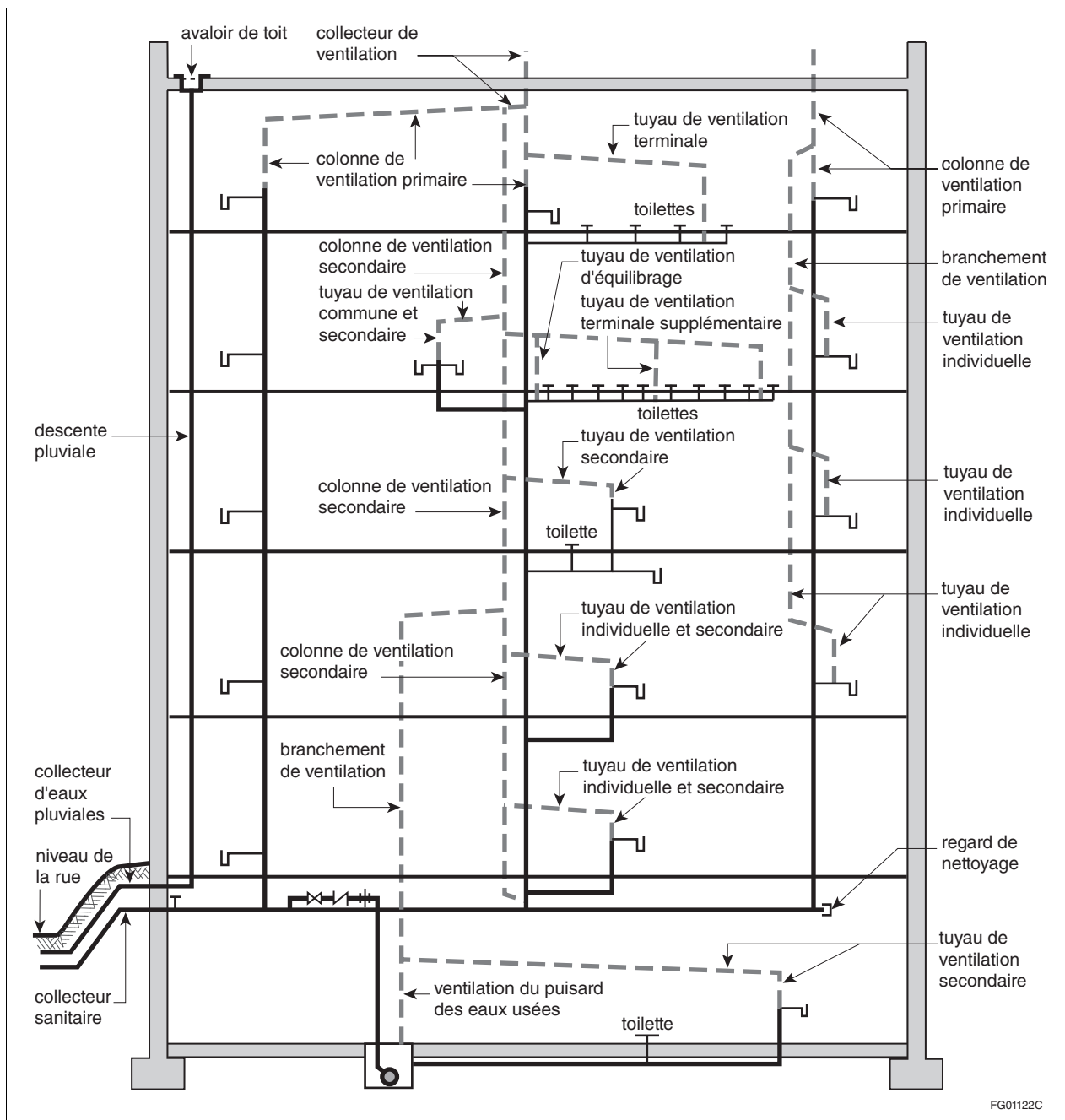
Figure A-1.4.1.2. 1)-I Réseau de ventilation
