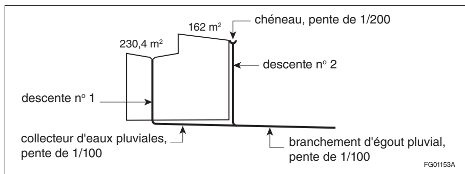
Figure 1-2 Réseau d'évacuation d'eaux pluviales (exemple 1, élévation)
