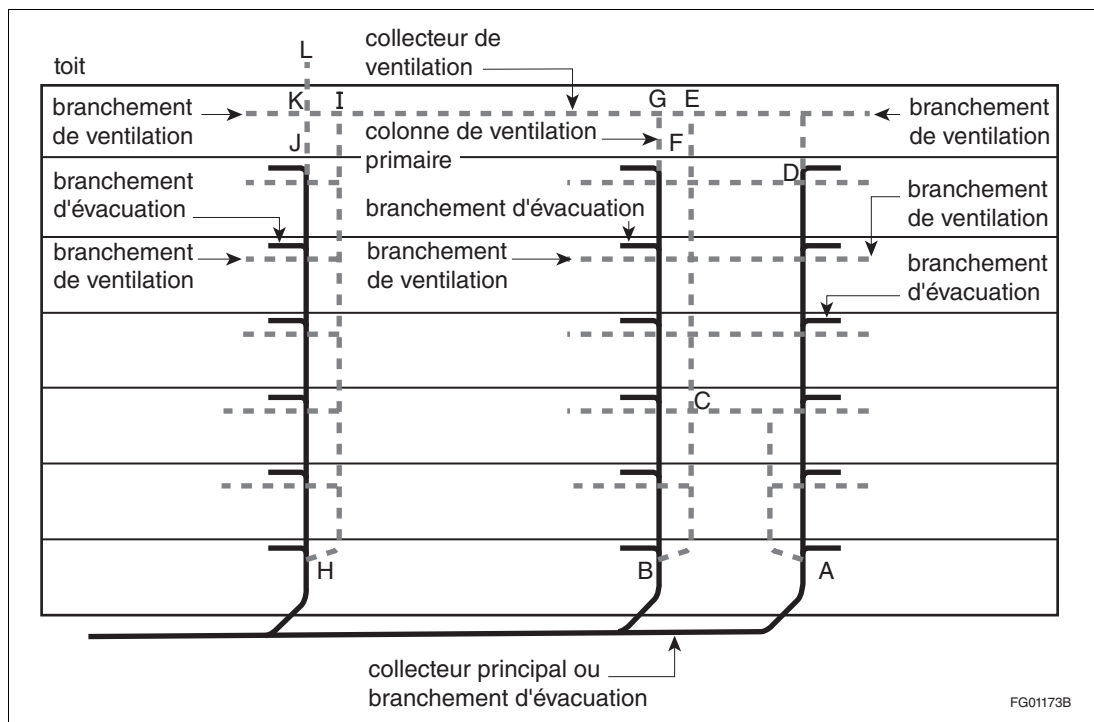
Figure A-2.5.8.3. et 2.5.8.4.-B
