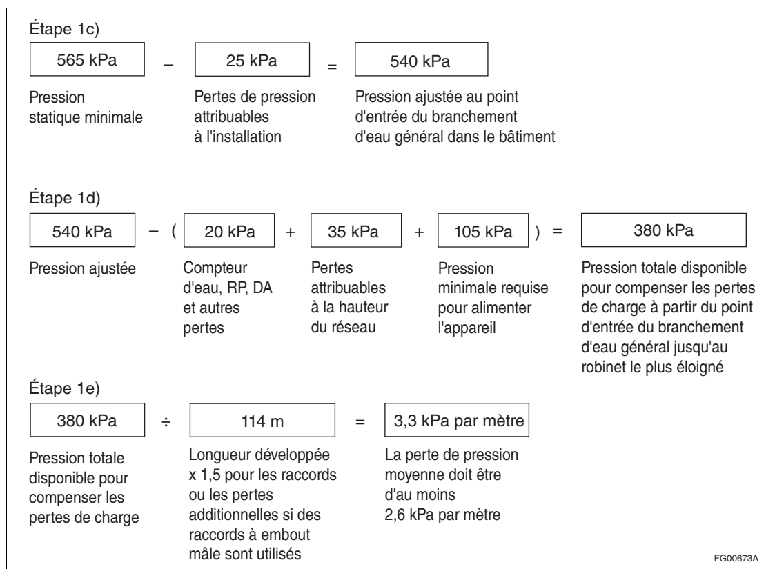
Figure A-2.6.3.1. 2)-B
