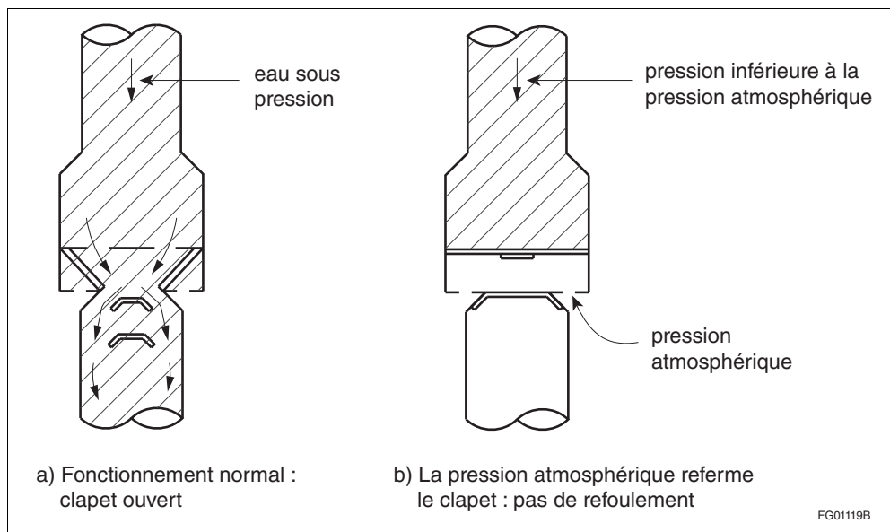
Figure A-1.4.1.2. 1)-B
