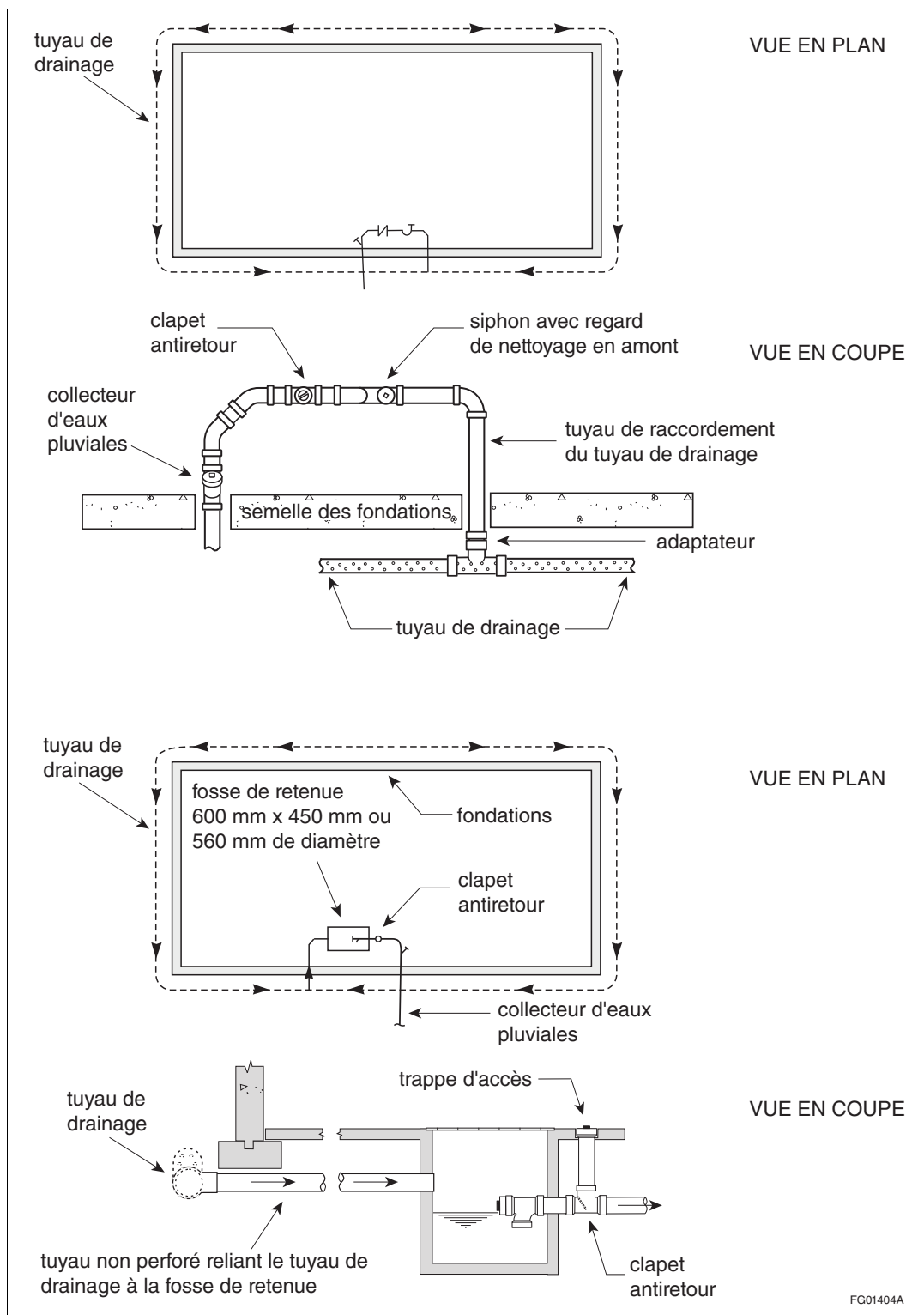
Figure A-2.4.5.3. 1) Raccordement d'un tuyau de drainage à un réseau d'évacuation
