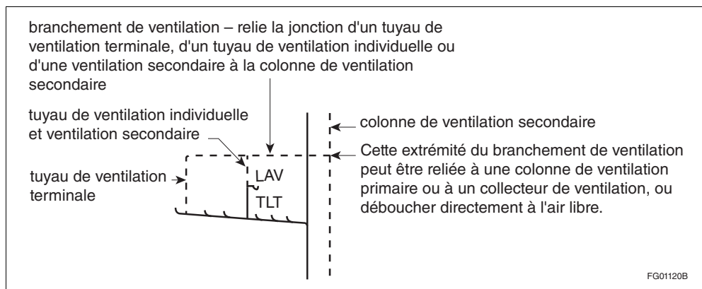
Figure A-1.4.1.2. 1)-A
