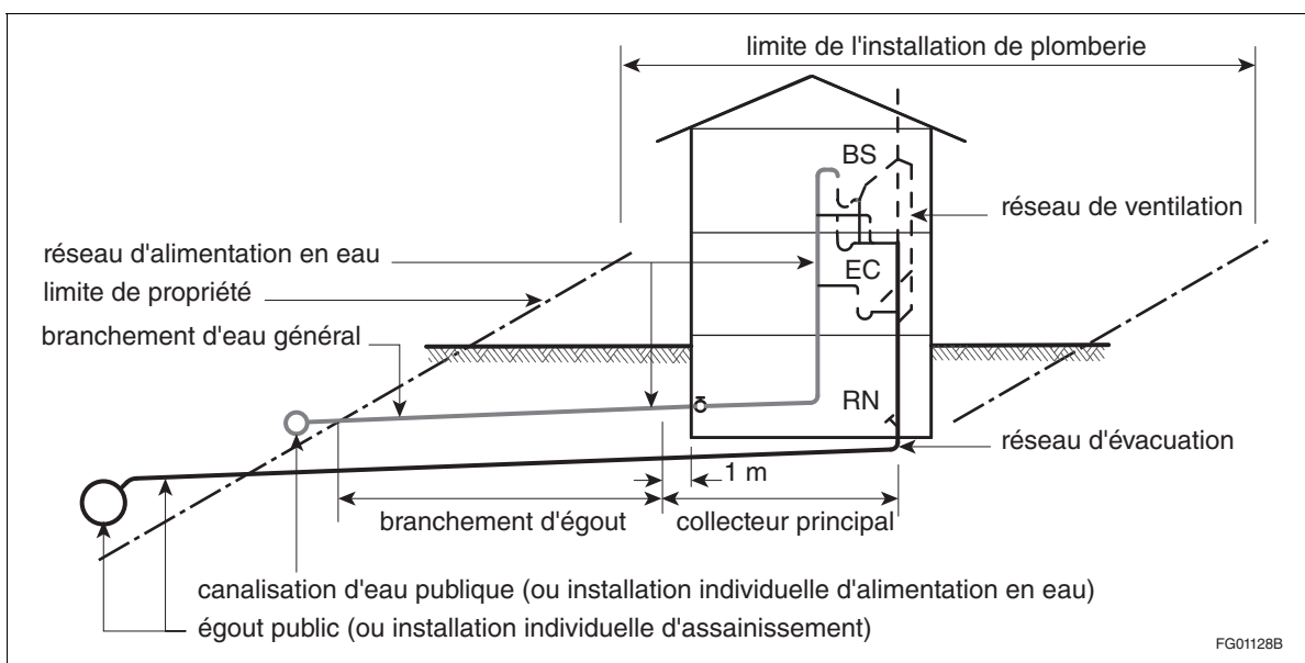
Figure A-1.4.1.2. 1)-G Installation de plomberie
