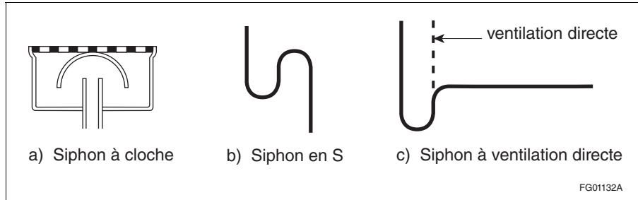
Figure A-2.2.3.1. 4) Types de siphon non permis
