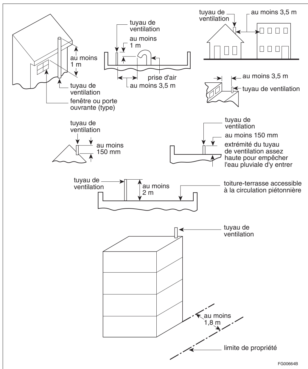
Figure A-2.5.6.5. 4) Extrémités supérieures des tuyaux de ventilation
