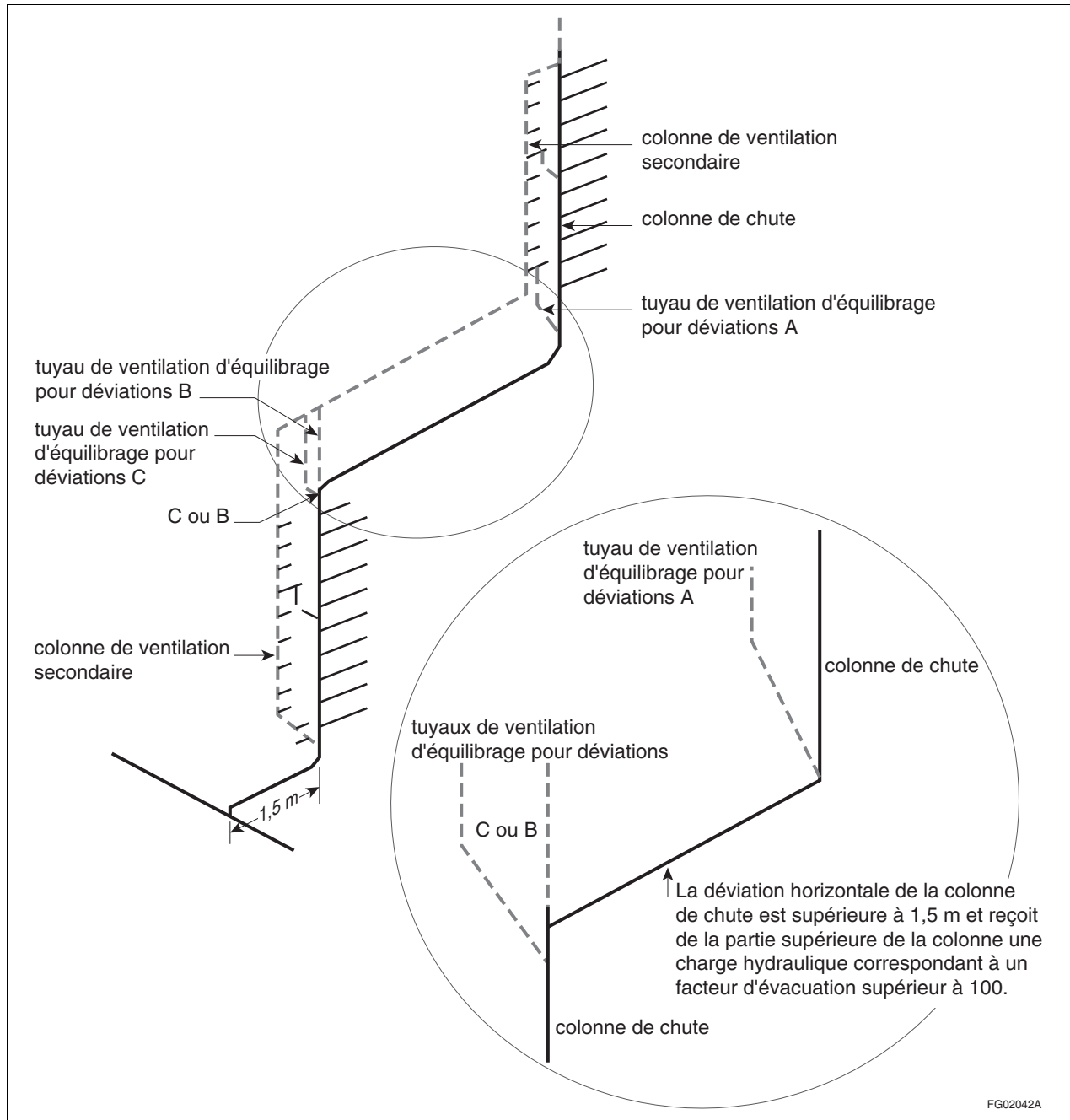
Figure A-2.5.4.4. 1) Tuyaux de ventilation d'équilibrage pour déviations
