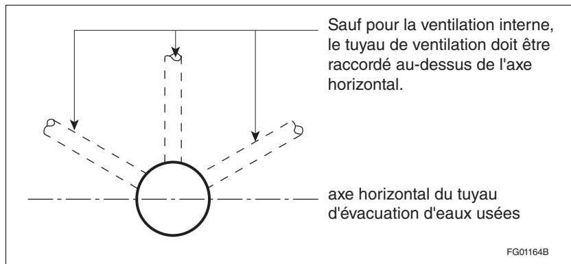
Figure A-2.5.6.2. 2) Raccordement des tuyaux de ventilation
