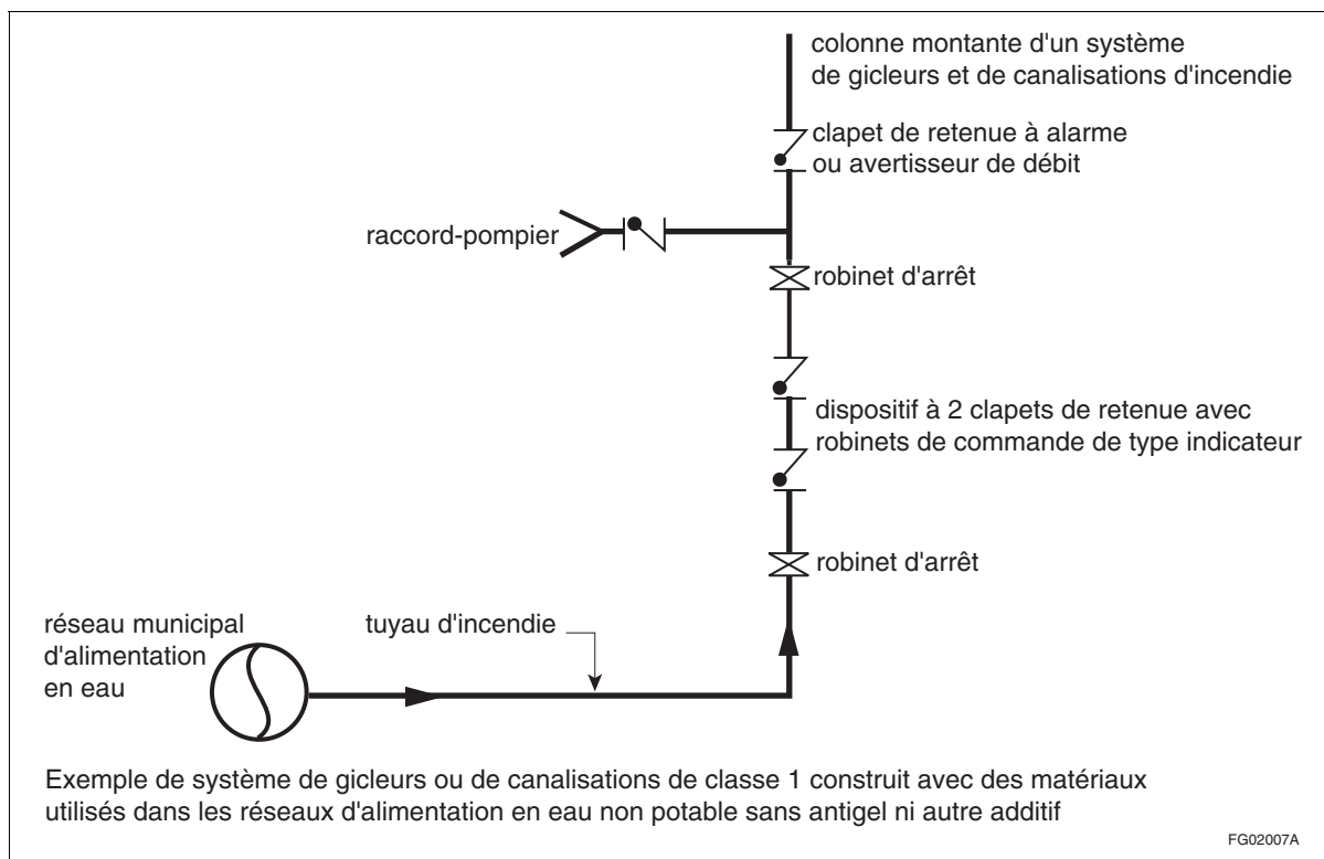
Figure A-2.6.2.4. 3) Raccordement du raccord-pompier et protection antirefoulement
