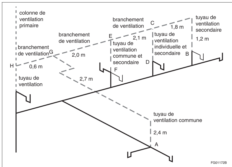
Figure A-2.5.8.3. et 2.5.8.4.-A
