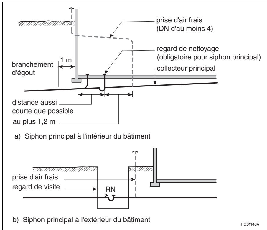
Figure A-2.4.5.4. 1) Emplacement des siphons principaux
