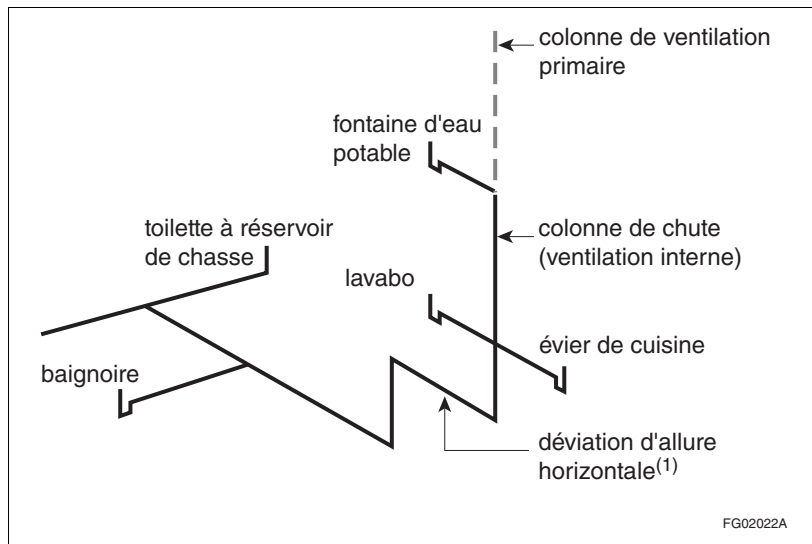
Figure A-2.5.2.1.-I Exemple de ventilation interne décrite à l'alinéa 2.5.2.1. 1)i)
