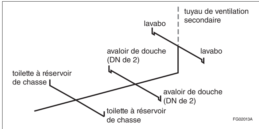
Figure A-2.5.2.1.-A Exemple de ventilation interne décrite à l'alinéa 2.5.2.1. 1)b)
