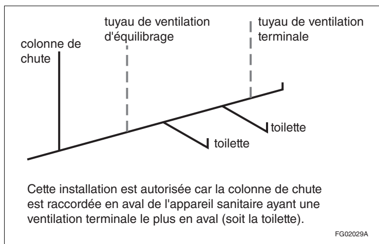
Figure A-2.5.3.1.-B Exemple de ventilation terminale décrite à l'alinéa 2.5.3.1. 1)c)
