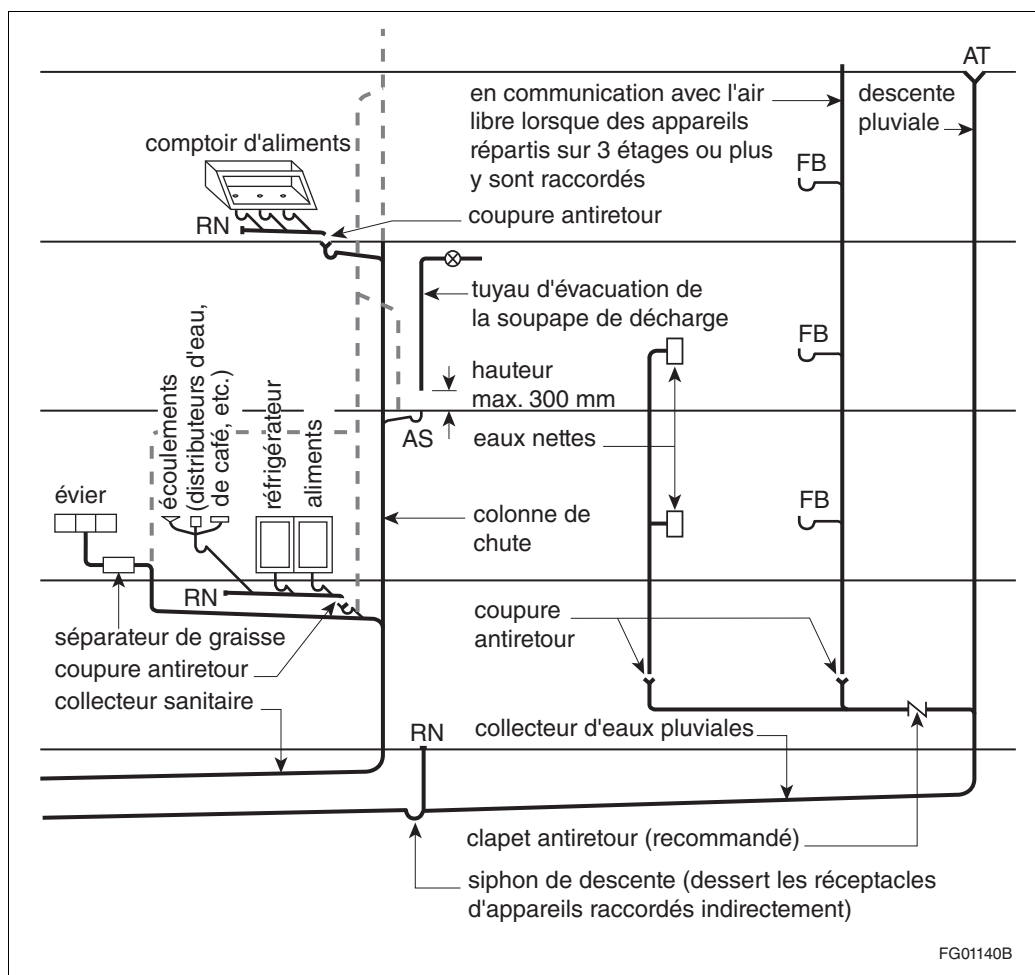
Figure A-2.4.2.1. 1)a)i) et e) Raccordements indirects
