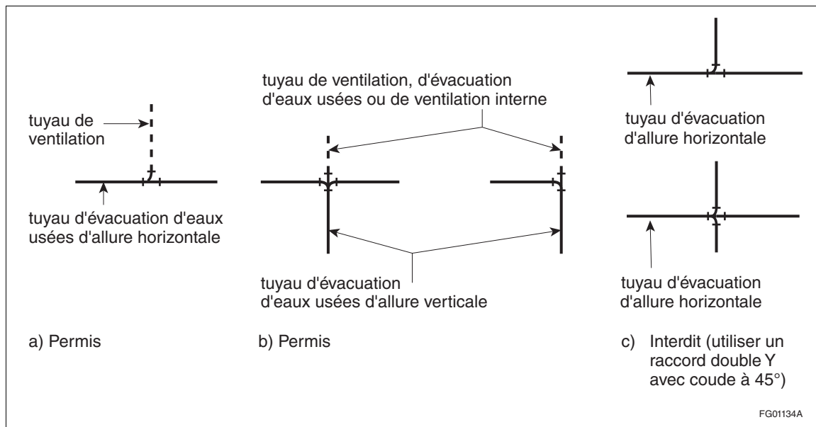
Figure A-2.2.4.2. Tés sanitaires dans les réseaux d'évacuation
