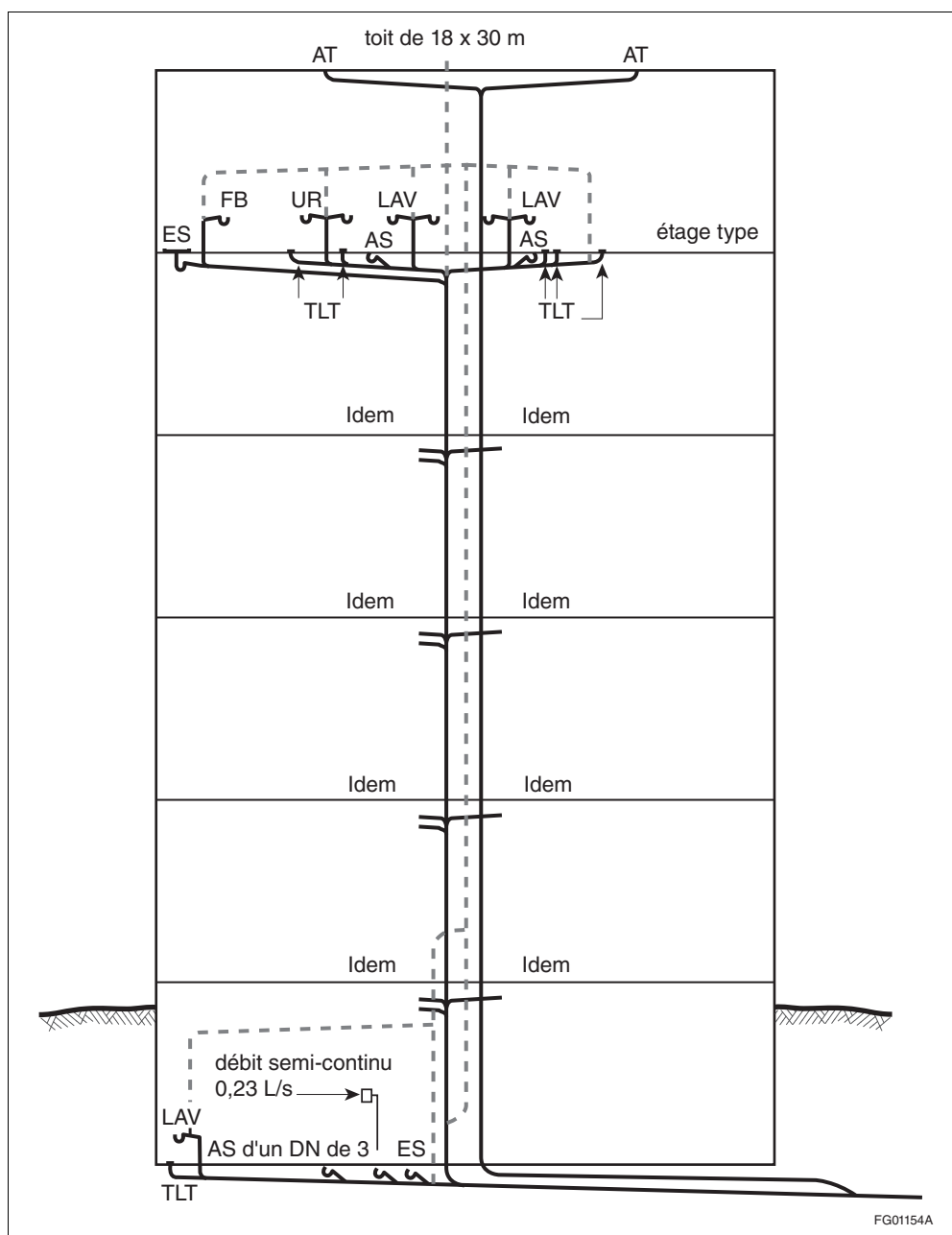
Figure 2-1 Réseau d'évacuation du bâtiment (exemple 2)
