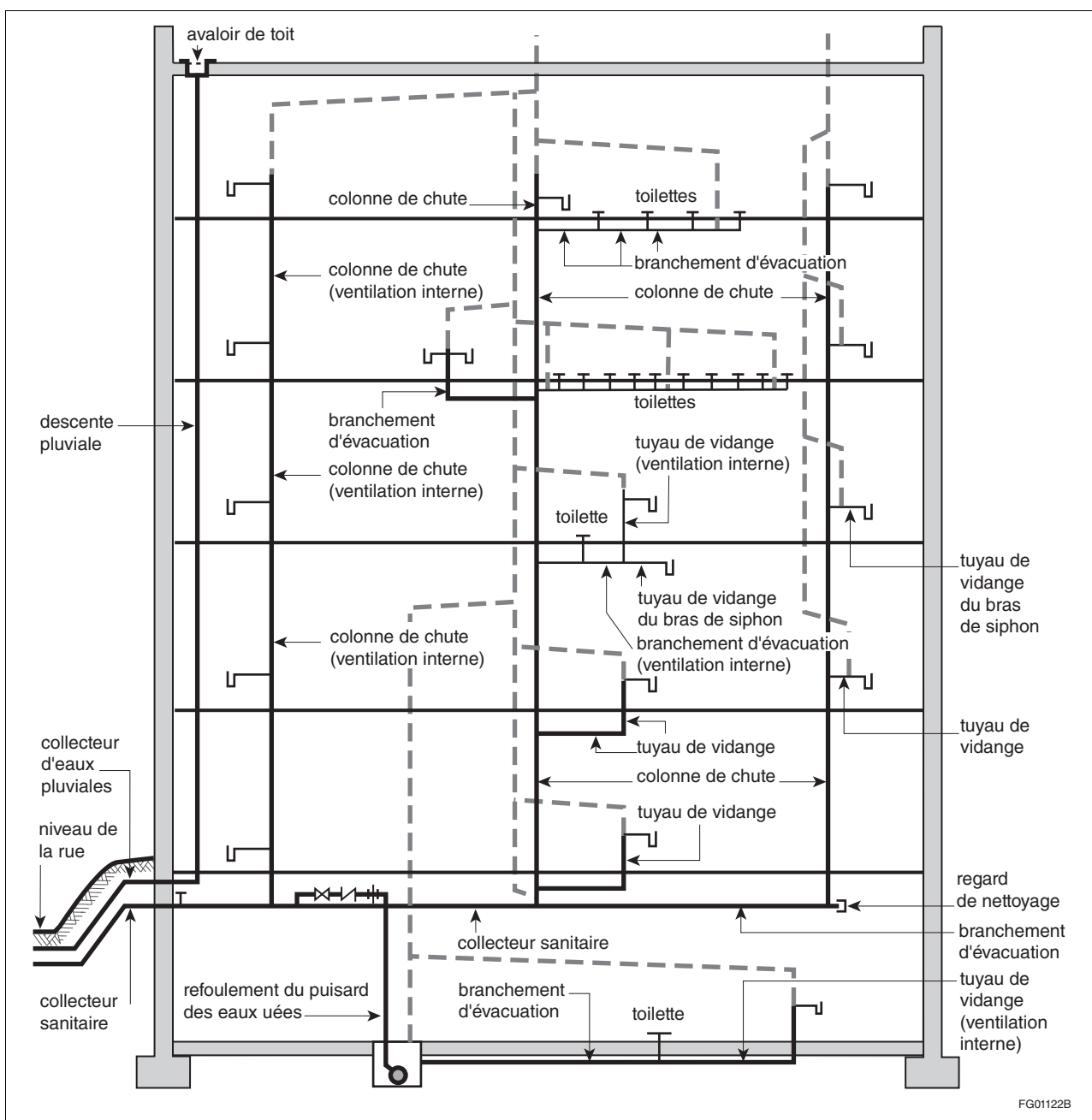
Figure A-1.4.1.2. 1)-H Réseau d'évacuation
