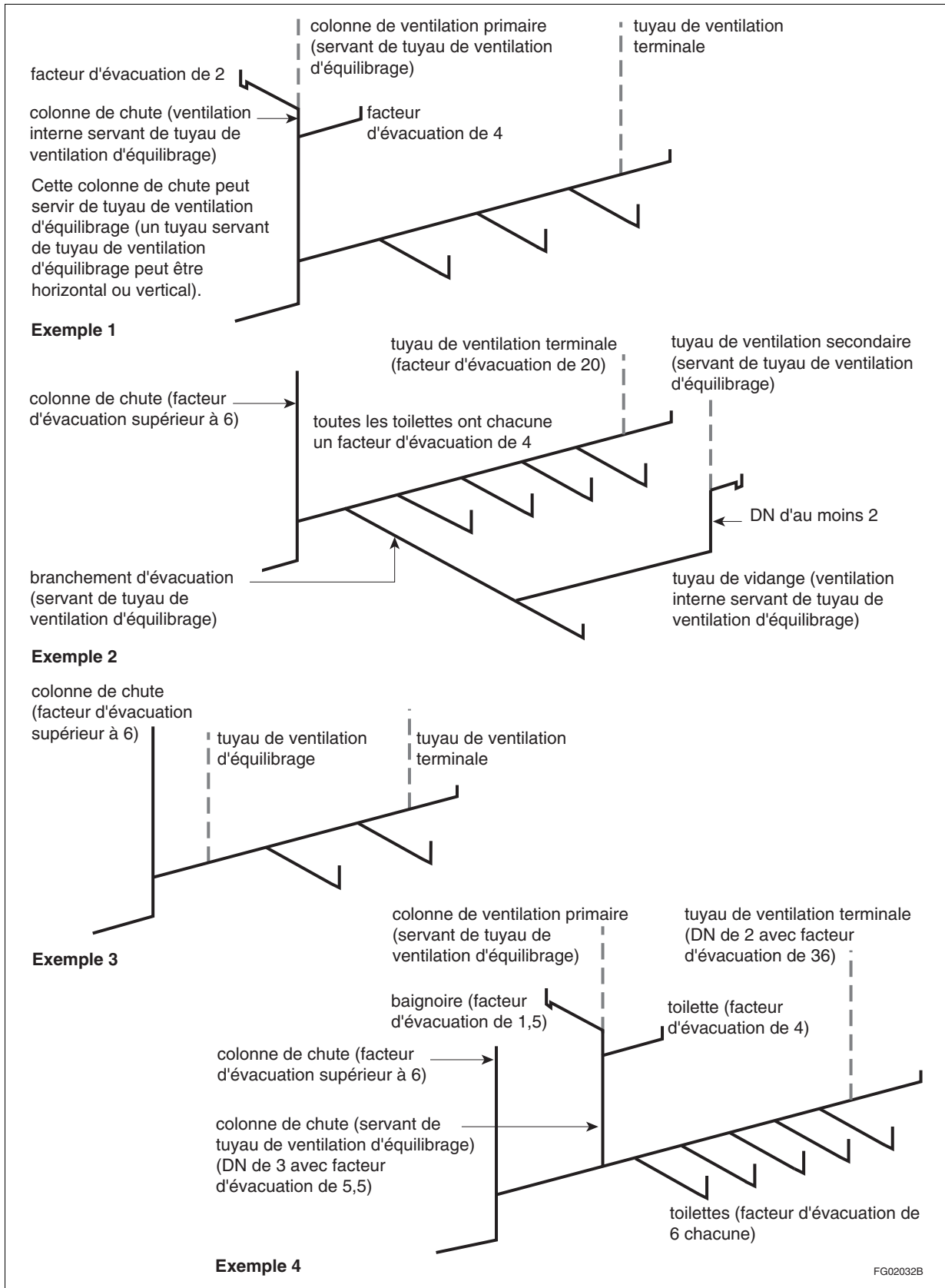
Figure A-2.5.3.1-E Exemple de ventilation terminale décrite au paragraphe 2.5.3.1. 4)
