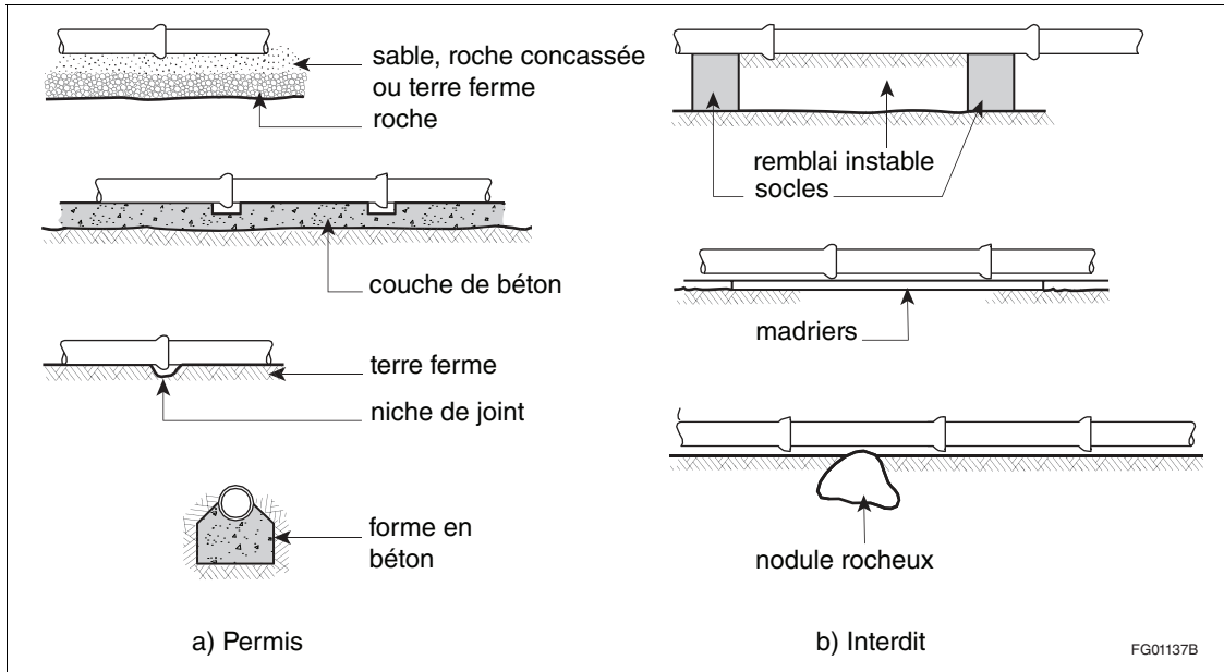
Figure A-2.3.4.6. 1) Support de la tuyauterie enterrée
