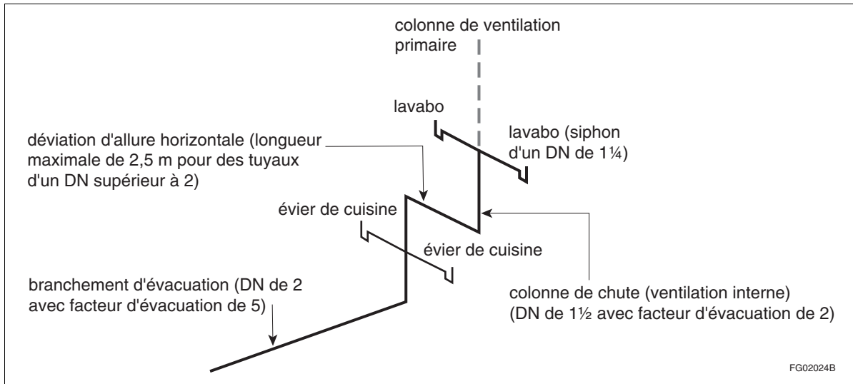
Figure A-2.5.2.1-K Exemple de ventilation interne décrite au sous-alinéa 2.5.2.1. 1)i)ii)
