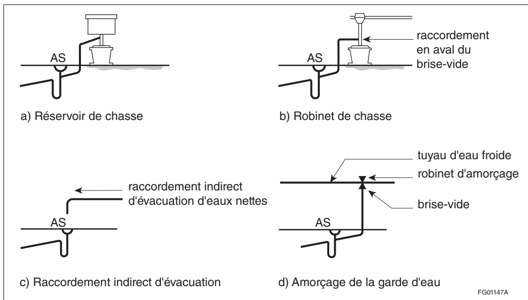
Figure A-2.4.5.5. 1) Maintien de la garde d'eau
