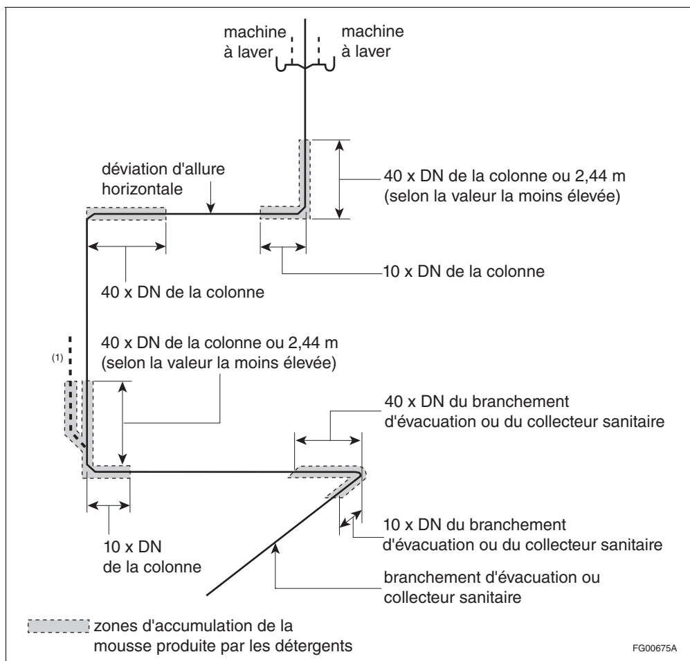
Figure A-2.4.2.1. 4) et 5) Zones de pression produites par la mousse
