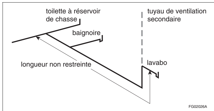
Figure A-2.5.2.1-M Exemple de ventilation interne décrite à l'alinéa 2.5.2.1. 1)k)
