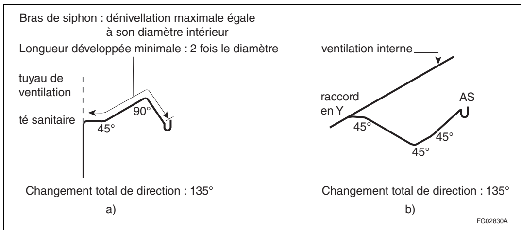
Figure A-2.5.6.3. 1)-B
