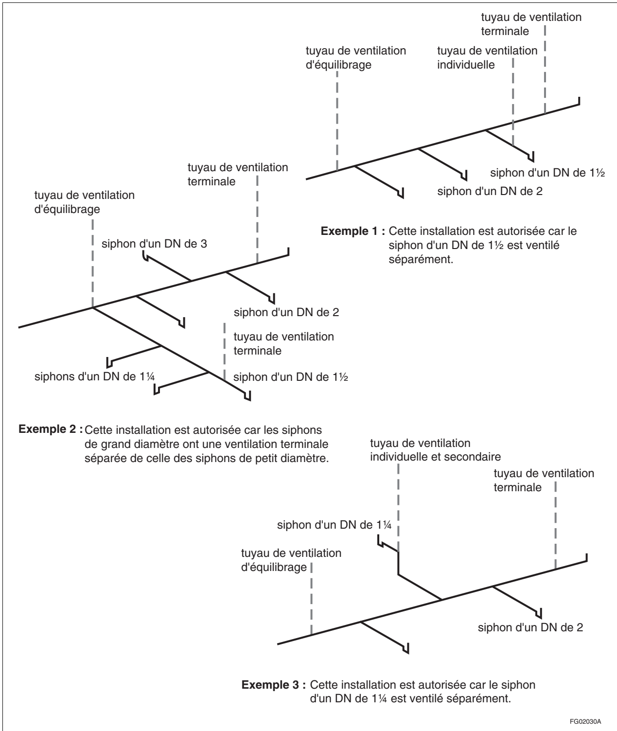
Figure A-2.5.3.1.-C Exemple de ventilation terminale décrite au paragraphe 2.5.3.1. 2) qui traite du DN des tubulures de sortie
