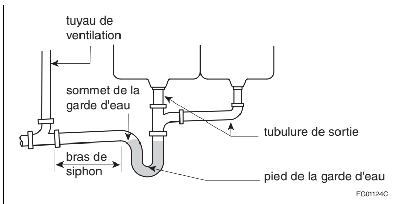
Figure A-1.4.1.2. 1)-K Bras de siphon et tubulure de sortie
