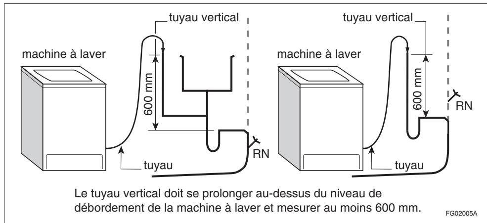
Figure A-2.4.9.3. 3) Illustration d'un tuyau vertical
