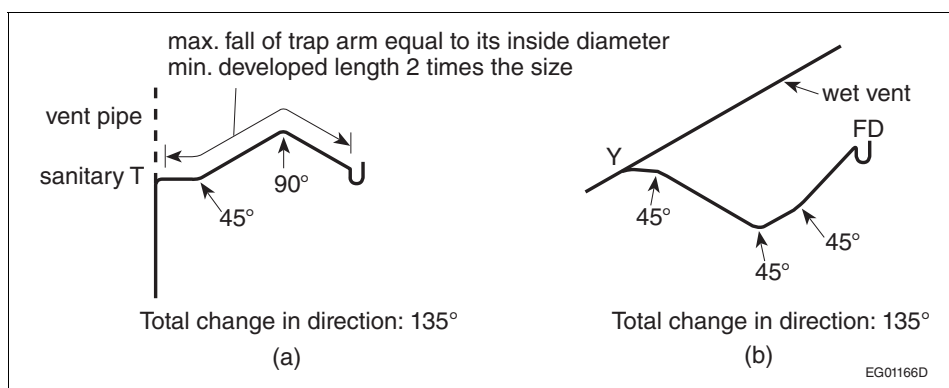
Figure A-2.5.6.3.(1)-B
