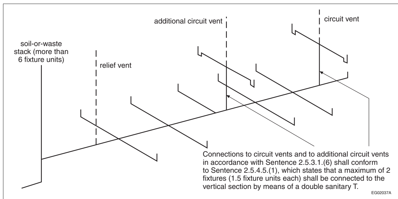
Figure A-2.5.3.1.-J
