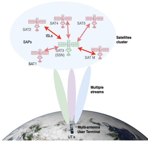
FIGURE 1. DM-MIMO scenario.
