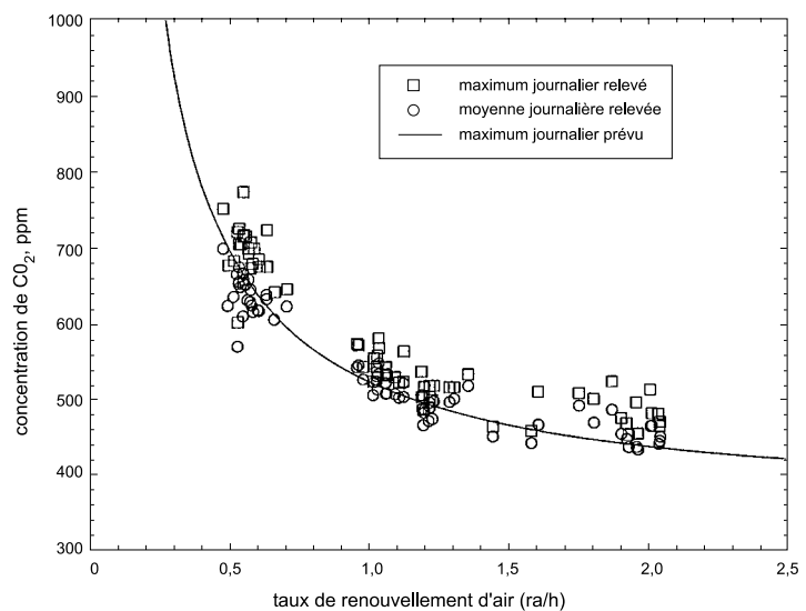
Figure 9. Comparaison entre les concentrations de CO_2 journalières maximales et moyennes à différents taux de renouvellement d'air
