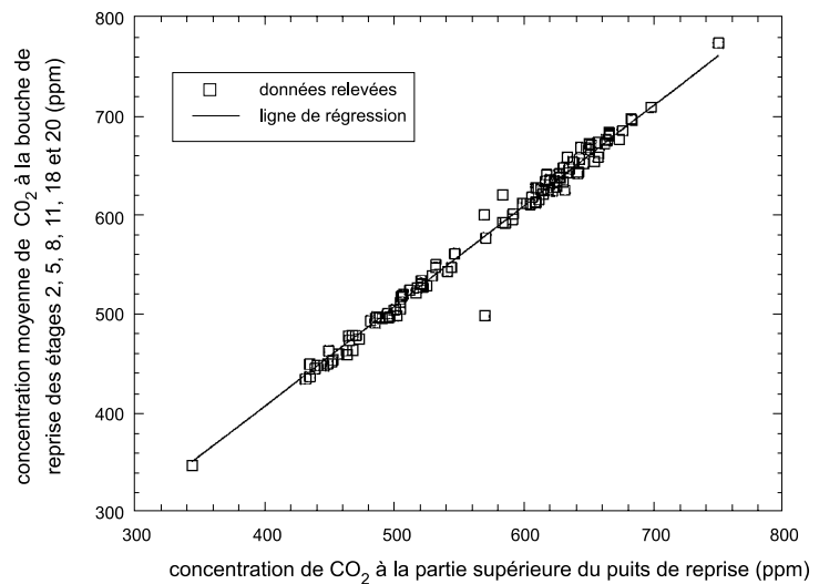
Figure 8. Comparaison entre les concentrations de CO_2 relevées à la partie supérieure des puits de reprise et celles mesurées aux bouches de reprise de chaque étage
