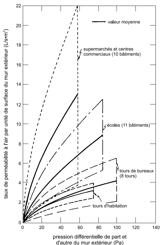
Figure 3. Mesures de l'étanchéité à l'air dans différents types de bâtiments
