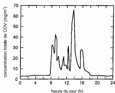
Figure 5. Concentration totale de COV dans un local abritant des photocopieuses
