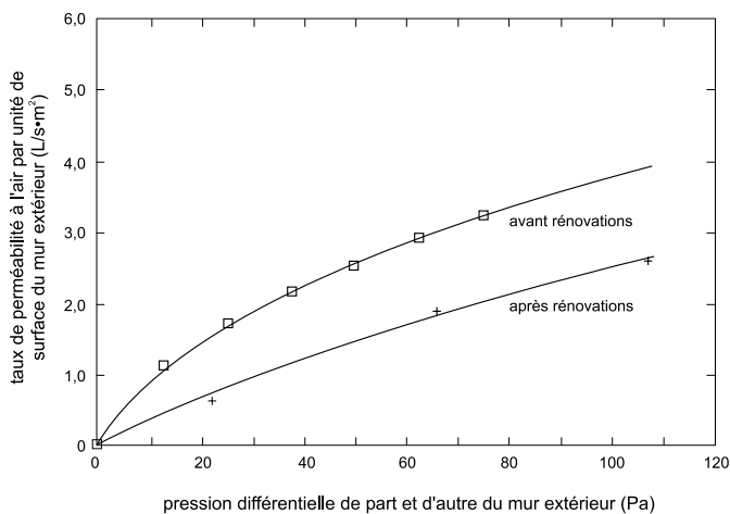
Figure 4. Mesures de l'étanchéité à l'air dans un immeuble de bureaux après rénovations
