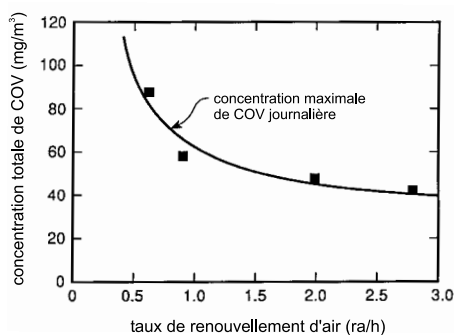
Figure 6. Capacité de dilution de l'air ventilé
