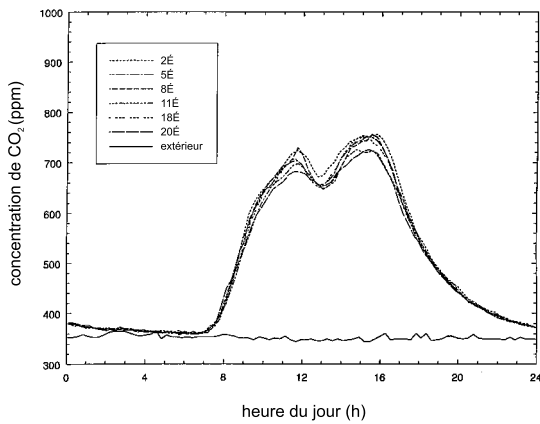
Figure 7. Concentrations types de CO_2 un jour de semaine, à différentes heures de la journée
