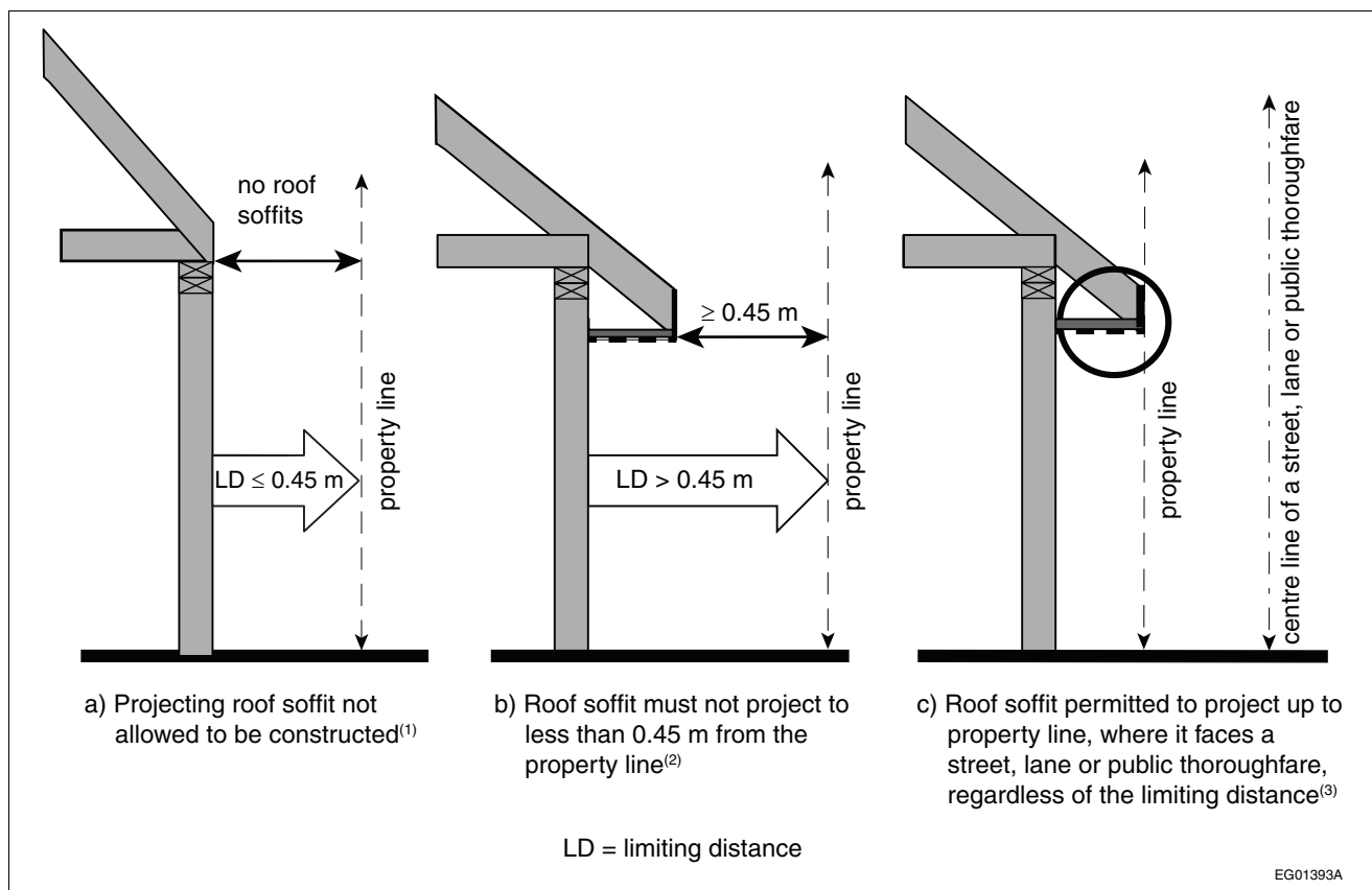
Figure A-9.10.14.5.(11) and 9.10.15.5.(10)
