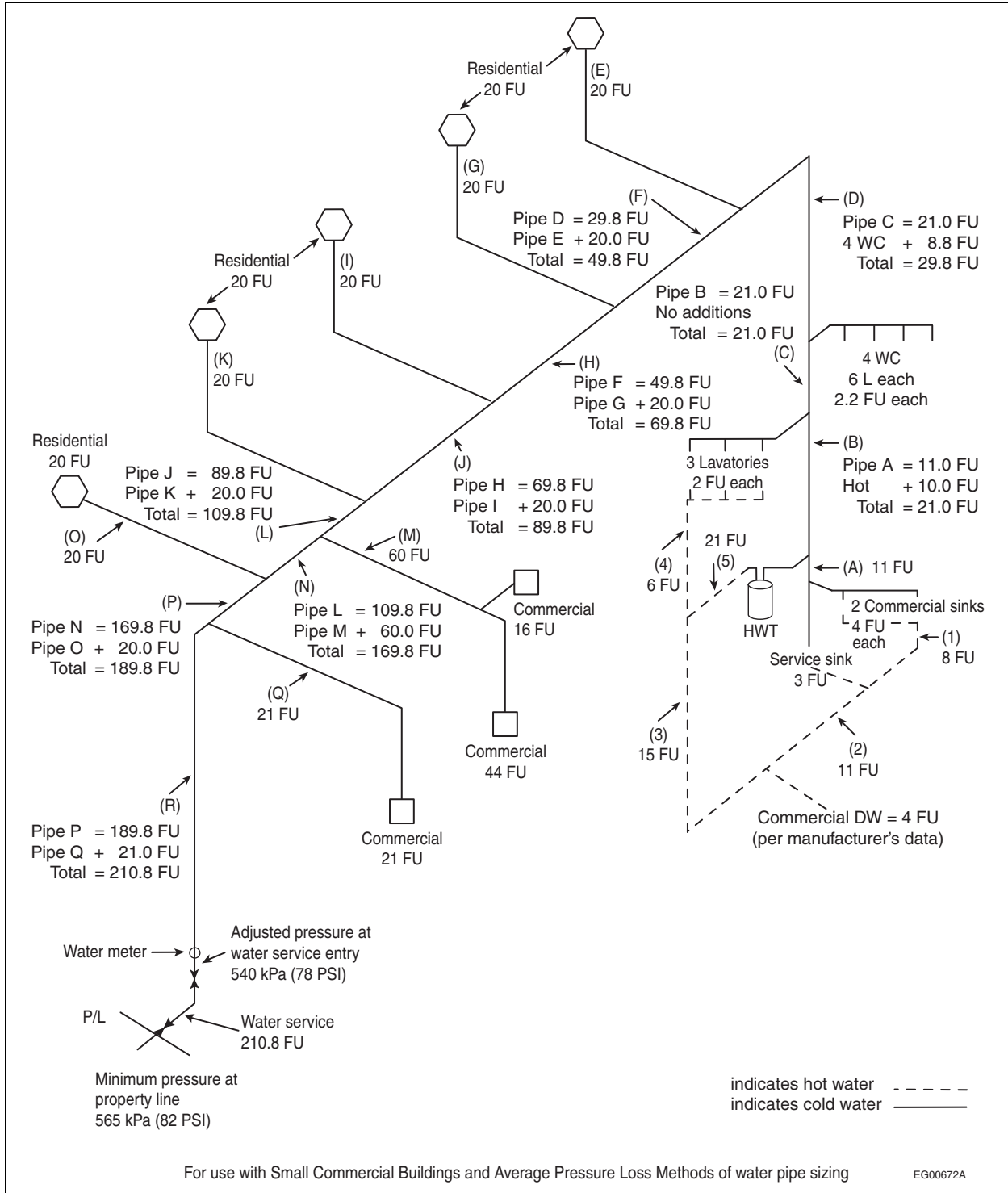
Figure A-2.6.3.1.(2)-A
